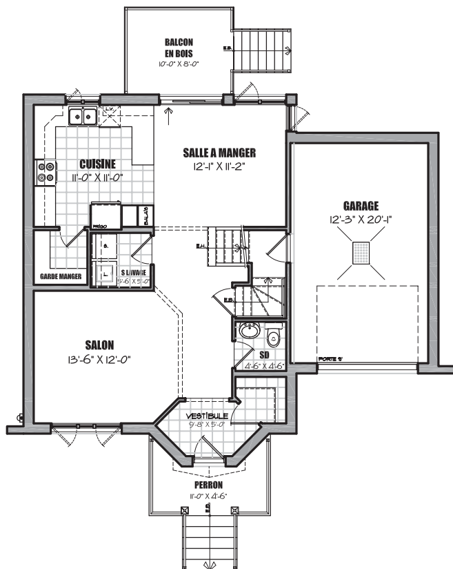
PLAN DU REZ-DE-CHAUSSÉE 38' L X 34' P
