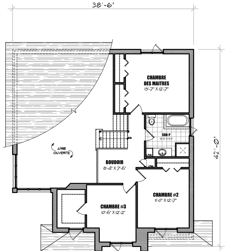
PLAN DE L'ÉTAGE 38,5' L X 42' P
