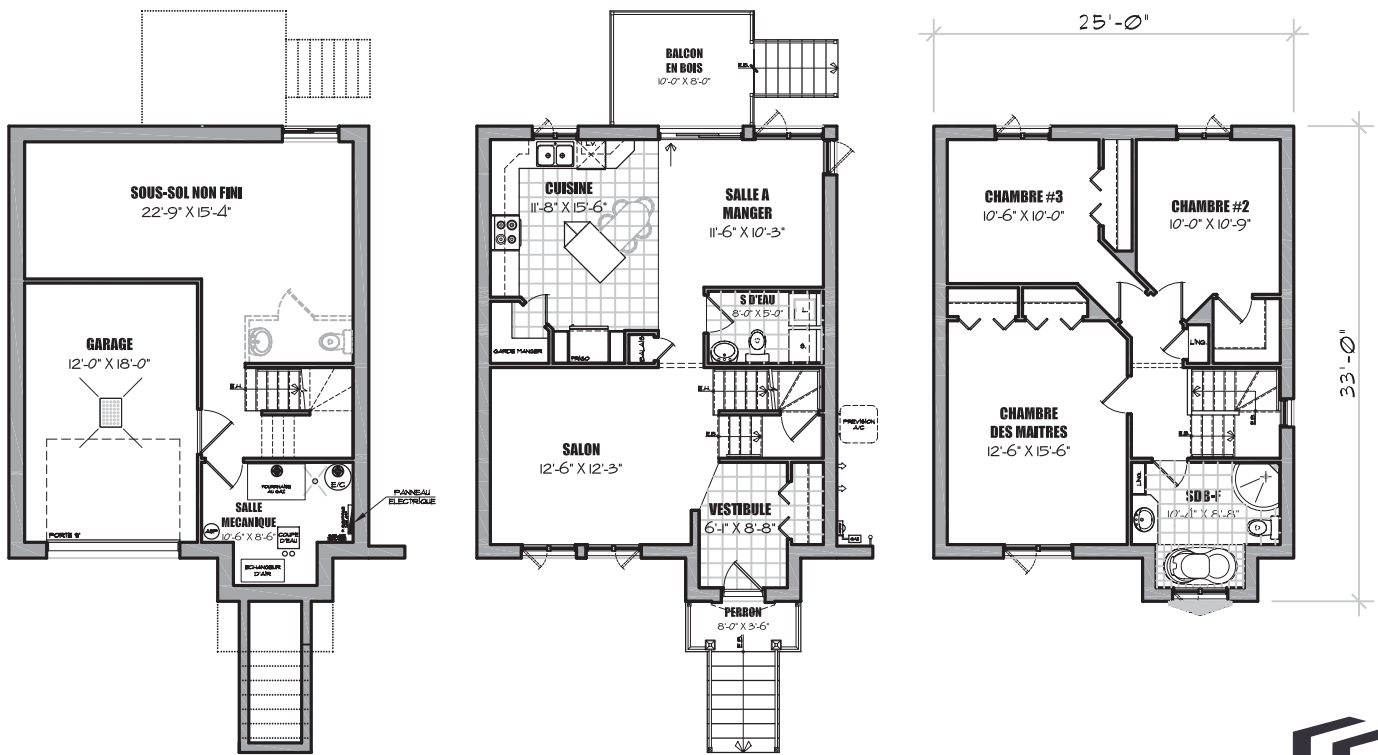
PLAN DU REZ-DE-CHAUSSÉE 25' L X 33' P
